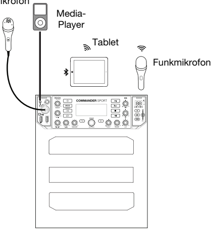
Vorderseite
