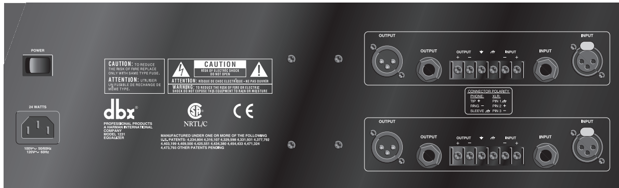
1215 - Correcteur graphique 15 bandes deux canaux
